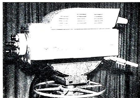
Bild 31. Drei-Röhren-Super-Orthikon-Farbkamera „TK41c“ der RCA
