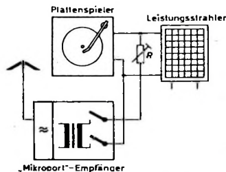
Bild 8. Schaltung zur Einblendung eines drahtlosen Mikrofons
