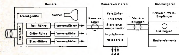
Bild 30. Geräteaufteilung einer Farbfernseh-Kameraanlage
