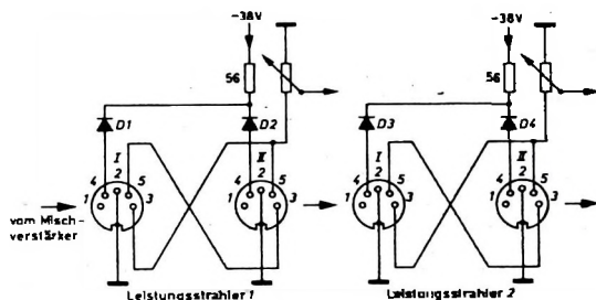
Bild 3. Eingangsschaltung des Leistungsstrahlers „VKL 303“
