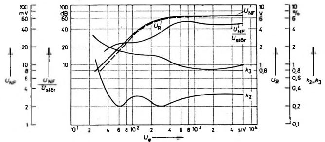
Bild 4. Meßkurven des FM-Teils; U_e ZF-Spannung an der Basis von T1, U_R Summenrichtspannung, U_{NF} NF-Spannung an 2,2 kOhm bei 1 kHz und 15 kHz Hub, U_{Stör}/U_{NF} AM-Störunterdrückung (FM: 120 Hz und 18 kHz Hub; AM: 1 kHz, m = 0,3 ), k_2 und k_3 Klirrfaktoren bei 120 Hz und 75 kHz Hub
