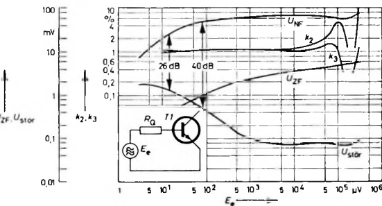
Bild 3. Meßkurven des AM-Teils; E_e Eingangsspannung an der Basis von T1 bei 1 MHz und 320 Ohm Quellwiderstand, U_{NF} NF-Spannung an 2,2 kOhm bei 1 kHz und m = 0,3 , U_{Stör} NF-Störspannung (Rauschen) an 2,2 kOhm, U_{ZF} ZF-Spannung an der Basis von T2, k_2 und k_3 Klirrfaktoren bei 1 kHz und m = 0,7
