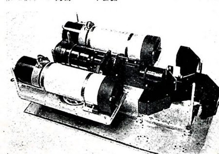
Bild 33. Anordnung von Variobjektiv, Farbteiler und Kameraröhren in der Drei-Röhren-Super-Orthikon-Farbkamera der Fernseh-GmbH
