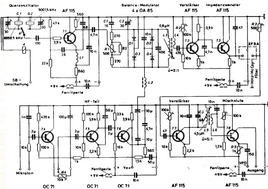
Bild 1. Schaltung des Exciters (SSB-Generator)
