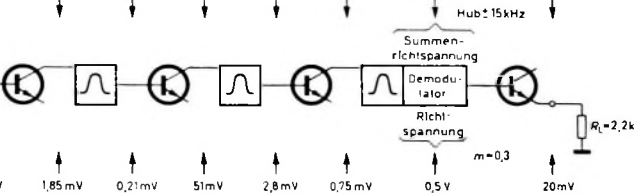
Bild 2. Pegeldiagramm für AM- und FM-Betrieb
