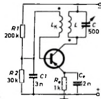
Bild 5. Meißner-Oszillator mit Transistor in Emitterschaltung
