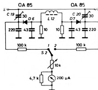
Bild 5. Schaltung der Stehwellenmeßbrücke
