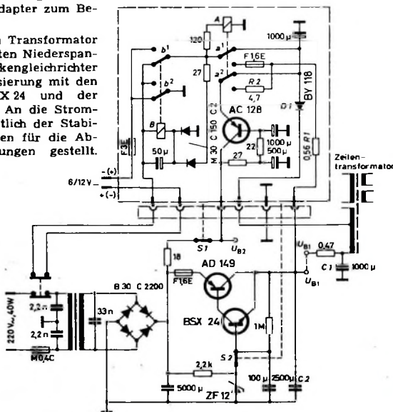
Bild 1. Schaltung des Netzsteils und Autoadapters im Fernsehgerät „Lady“ von Graetz (Relaisstellung 6 V-, Minuspol an Masse)
