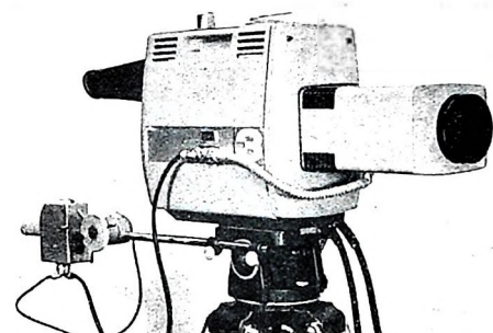
Bild 34. Drei-Röhren-Plumbikon-Farbkamera von Philips
