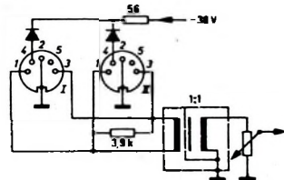
Bild 3. Eingangsschaltung des Leistungsstrahlers „VKL 303“
