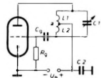
Bild 7. Induktiver Dreipunktschaltung mit Reihenspeisung
