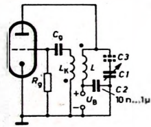
Bild 3. Meißner-Oszillator mit Reihenspeisung, bei dem der Abstimmkondensator nicht unter Anodenspannung steht
